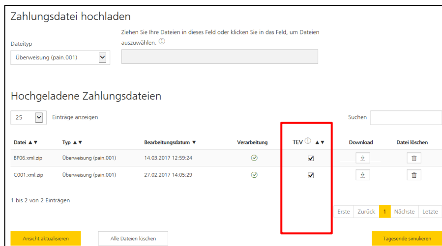
Abbildung 5: Tagesendverarbeitung simulieren
